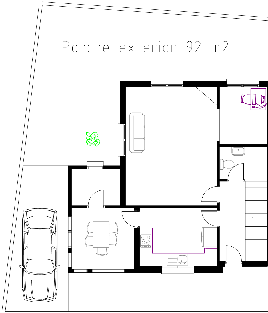
PLANTA baja 72 M2
